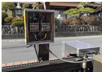
【写真2】 駆動モーターと配電盤
